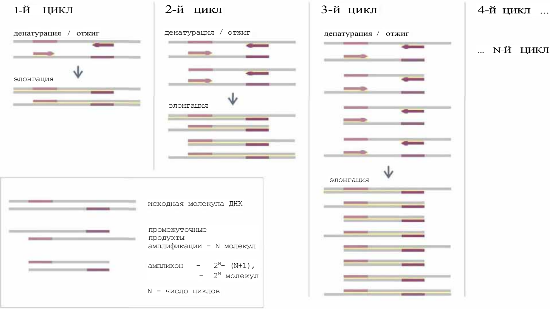
Рис.2. Накопление продуктов амплификации.
