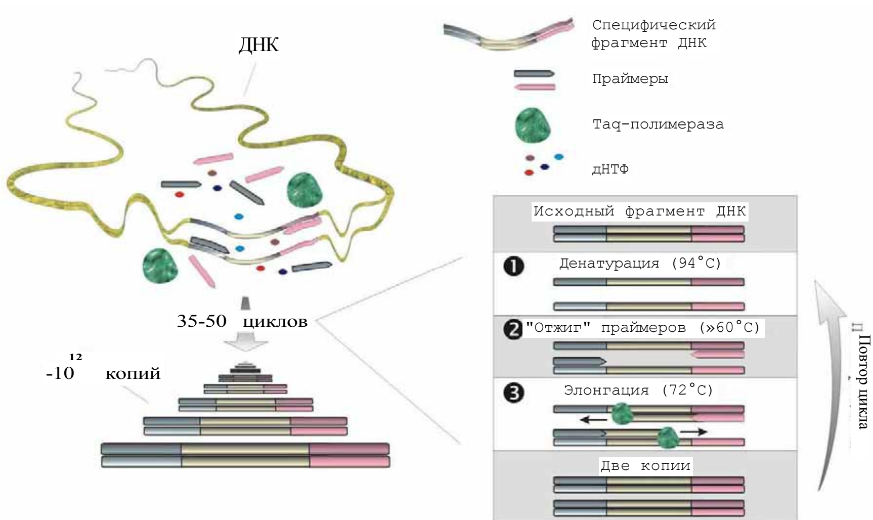
Рис.3. Принцип полимеразной цепной реакции.
